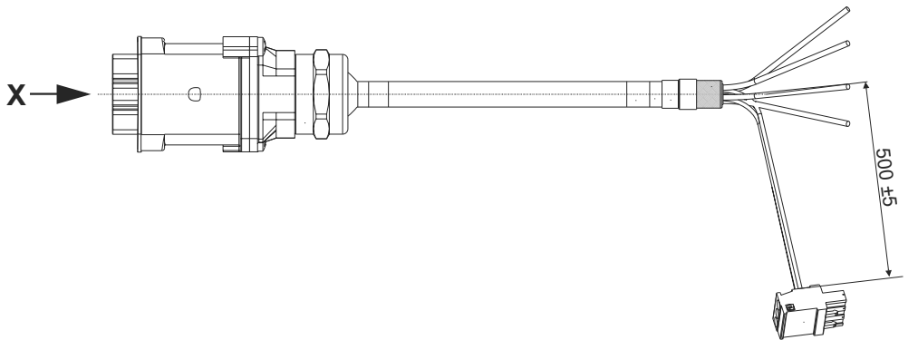
Bild 33: Bremsmotorkabel CFM
