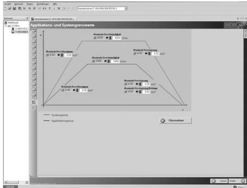
Bild 15: Applikations- Systemgrenzwerte
