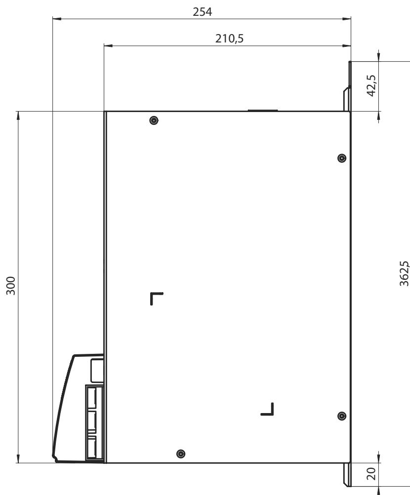
Bild 23: Abmessungen 24-V-Schaltnetzteilmodul
