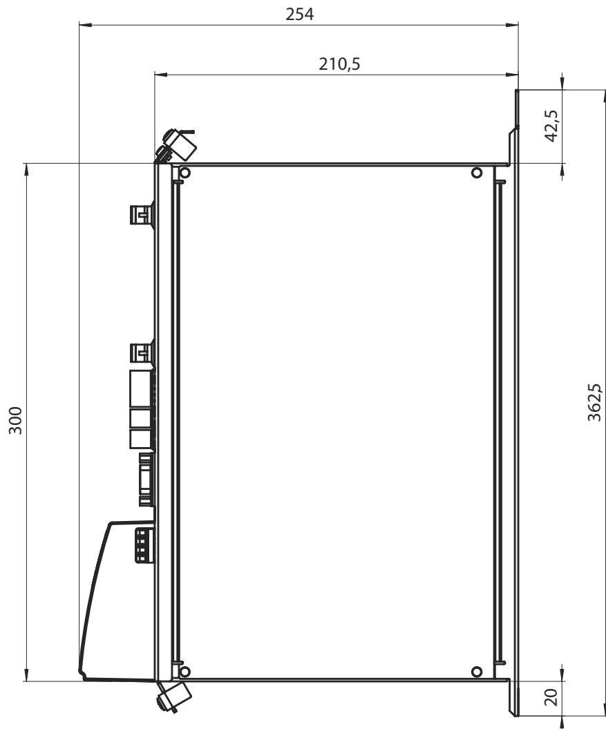
Bild 22: Abmessungen Mastermodul
